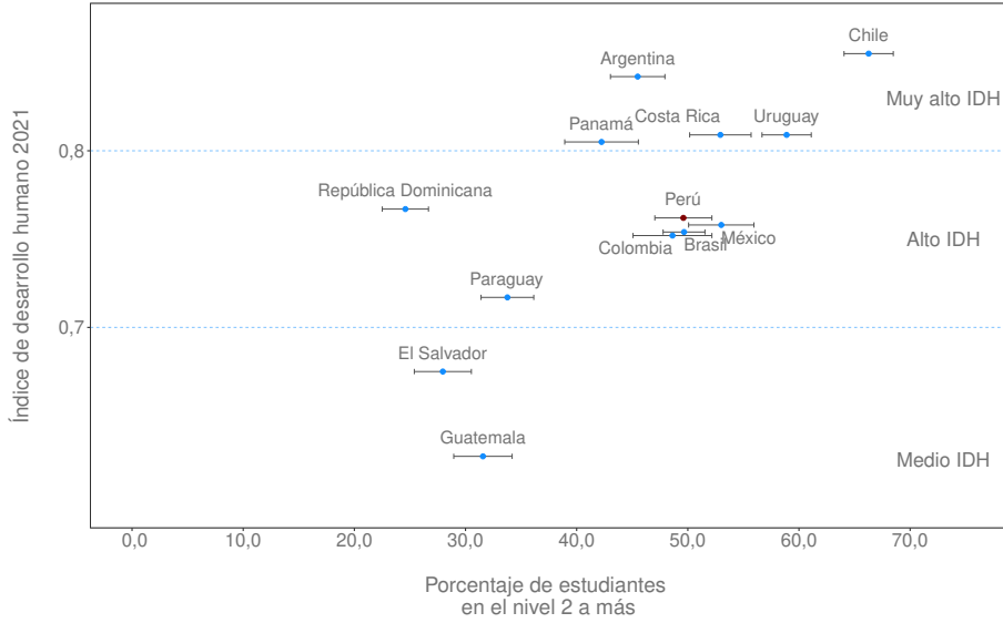
Figura G.1.1 Relación entre el IDH y el porcentaje de estudiantes que alcanzan o superan el nivel 2 en Lectura
